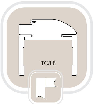
Telaio tondo con coprifili lisci (disponibile solo per porte con vetro)
