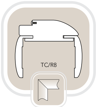
Telaio tondo con coprifili tondi (disponibile solo per porte con vetro)
