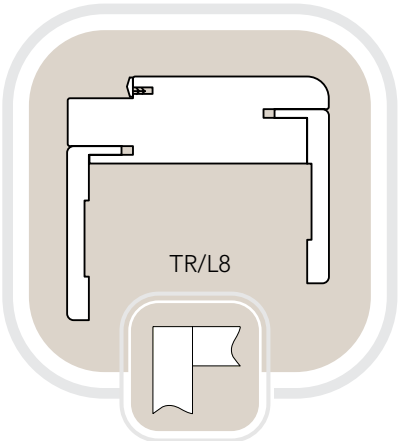
Telaio lineare con coprifili lisci
